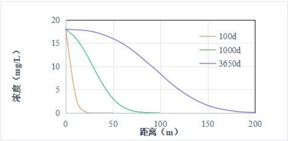
图 5.2-2 发生泄漏后石油类污染物浓度变化趋势图（情景 1）
