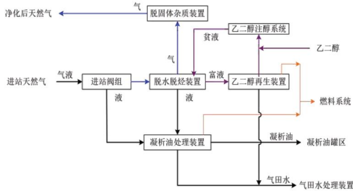
图 3.3-6 克深天然气处理厂工艺流程图
