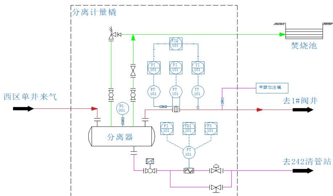
图 3.3-4 克深 31 分水站工艺原理流程图
