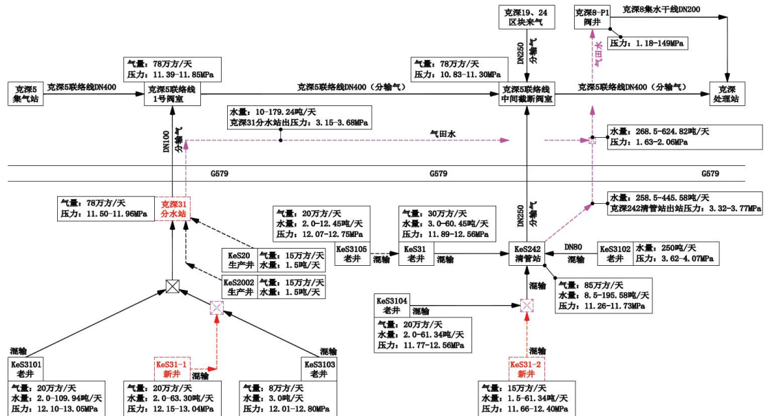
图 3.3-2 克深 31 区块总体流向示意图
