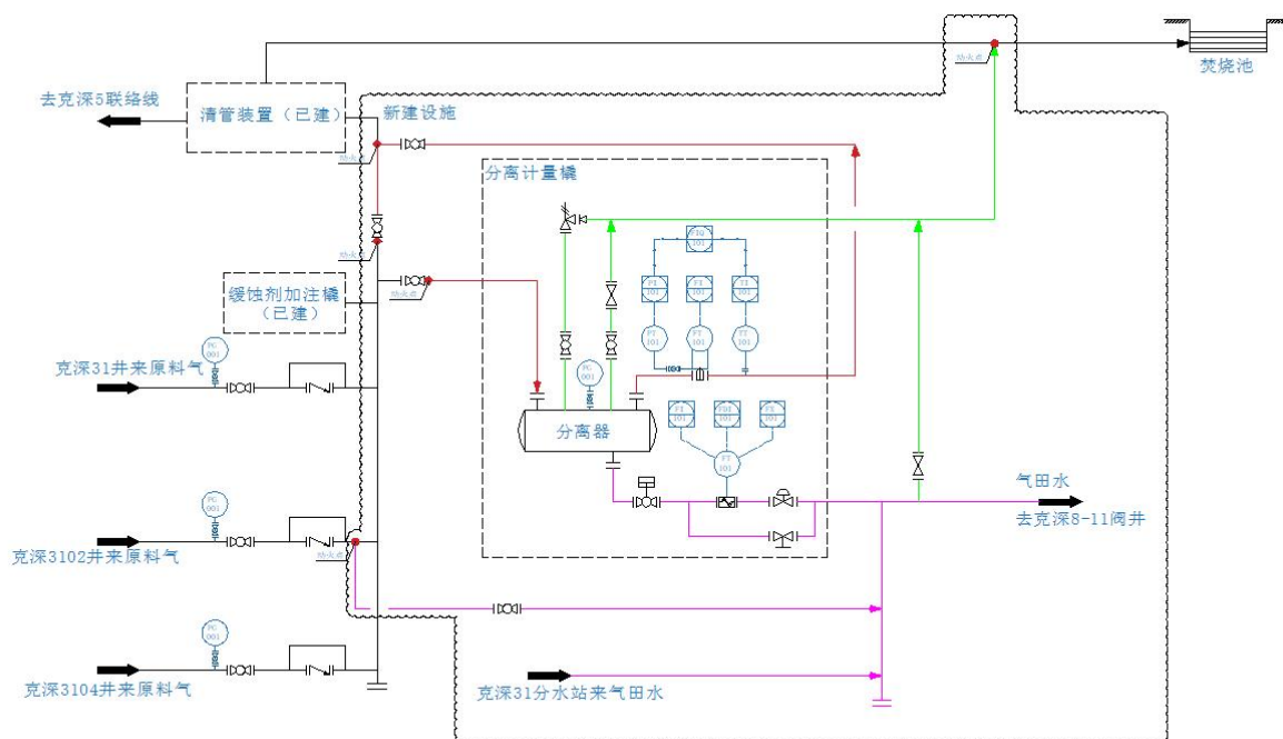
图 3.3-5 克深 242 清管站改造工艺原理流程图
