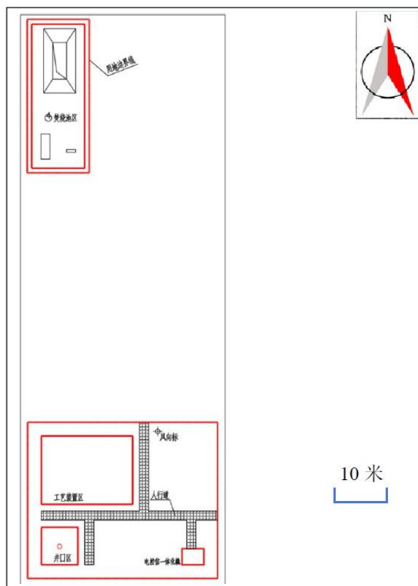
图3.2-1 井场平面布置示意图
